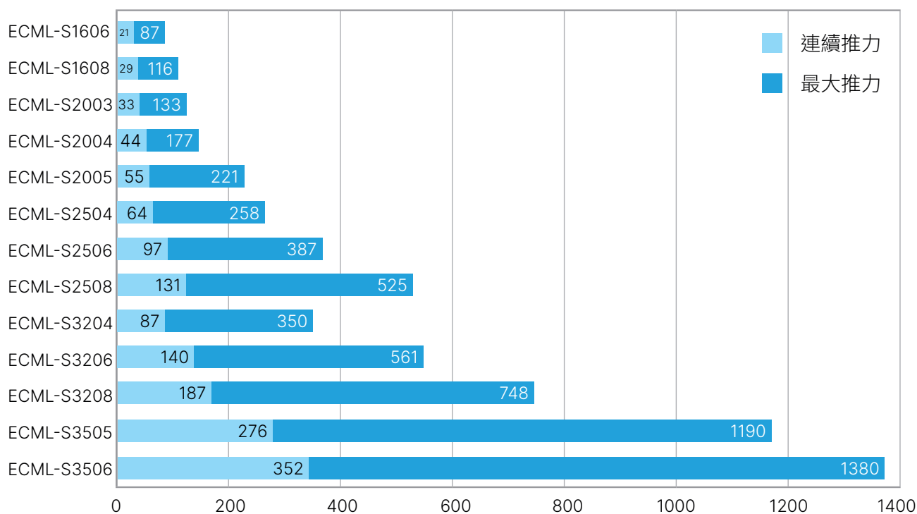
推力表 (N)
