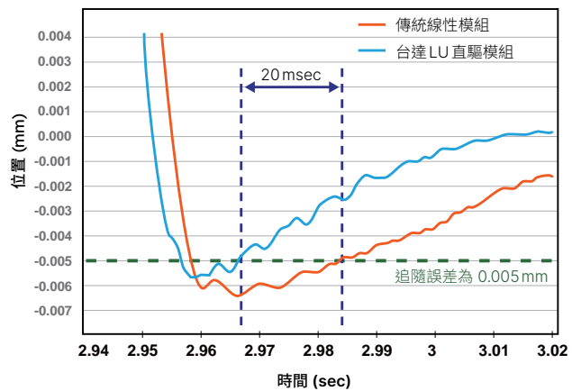
雷射干涉儀量測結果
