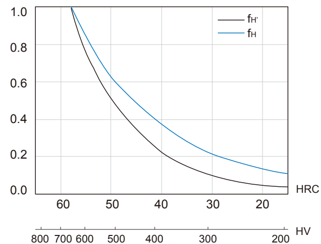
圖31. 硬度係數
