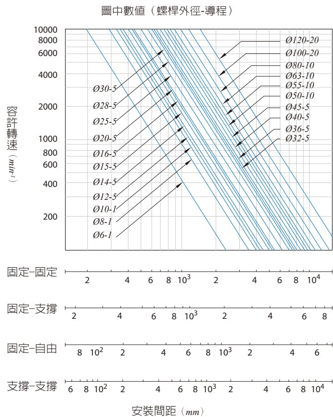
圖10. 容許轉速圖表
