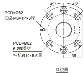
D 視圖
