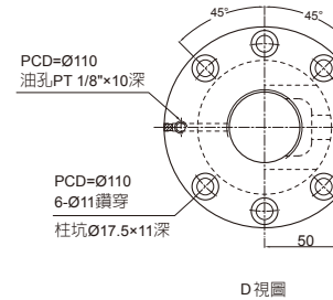
D 視圖
