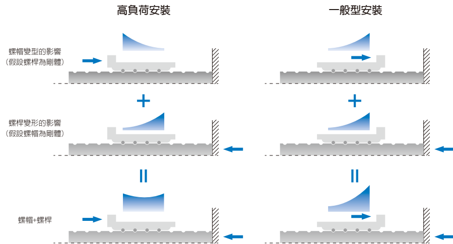
圖8. 負載分布圖
