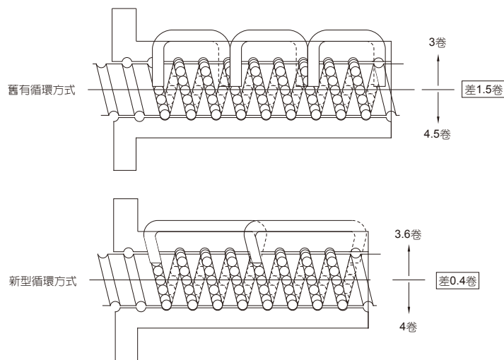
圖4. 高負荷螺桿新舊循環圈數差異比較
