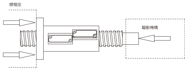
圖7. 高負荷螺桿建議安裝方式
