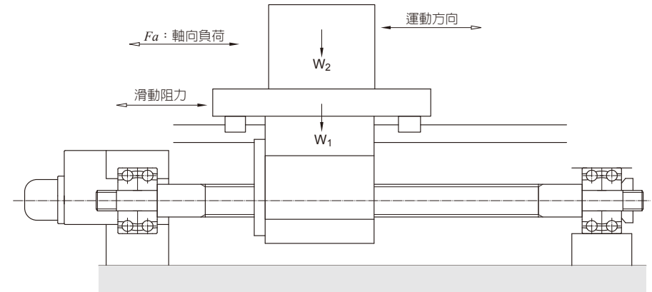
圖15. 水平搬運裝置簡圖
