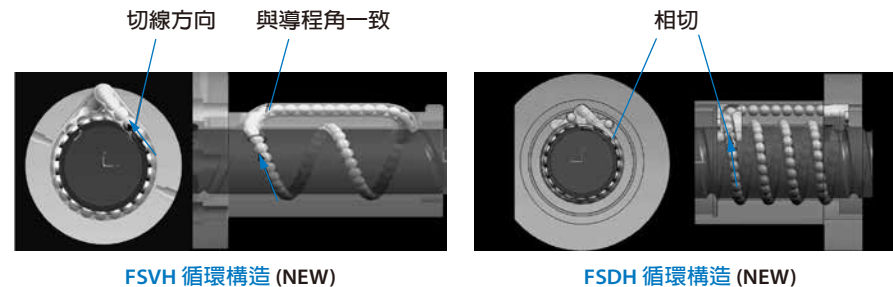
圖5. FSVH、FSDH 循環構造
