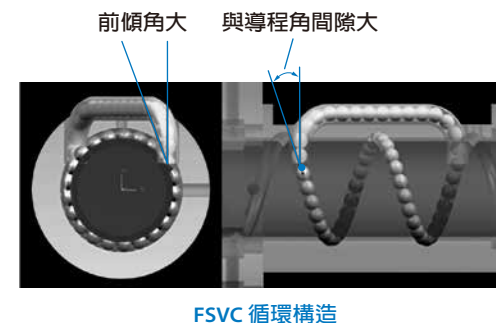
圖6. 舊型式 FSVC 循環構造
