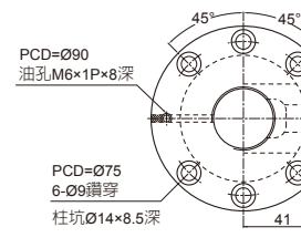
D 視圖
