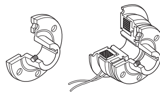
1 型电枢
