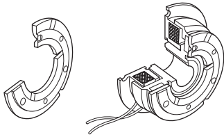
3 型电枢
