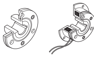
2 型电枢
